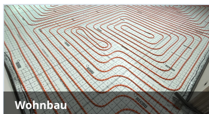
Zuleitungen in der Dämmebene
